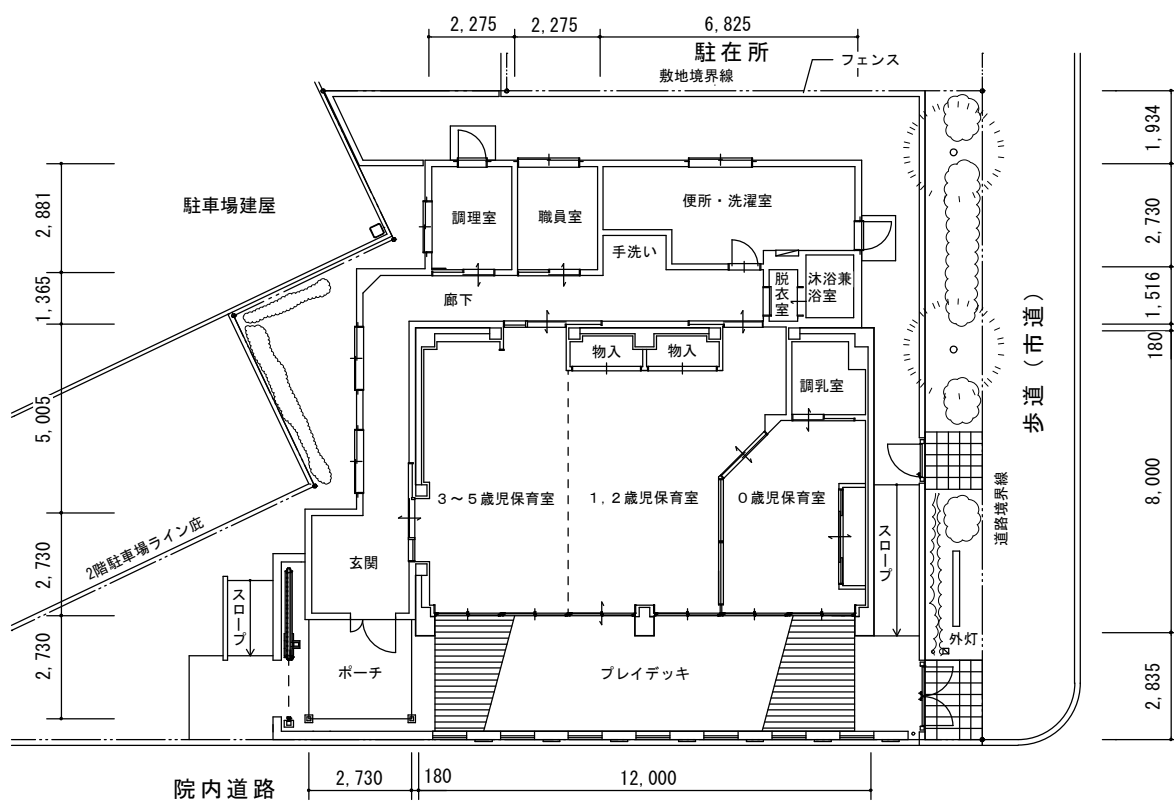
平面図 S=1/200
