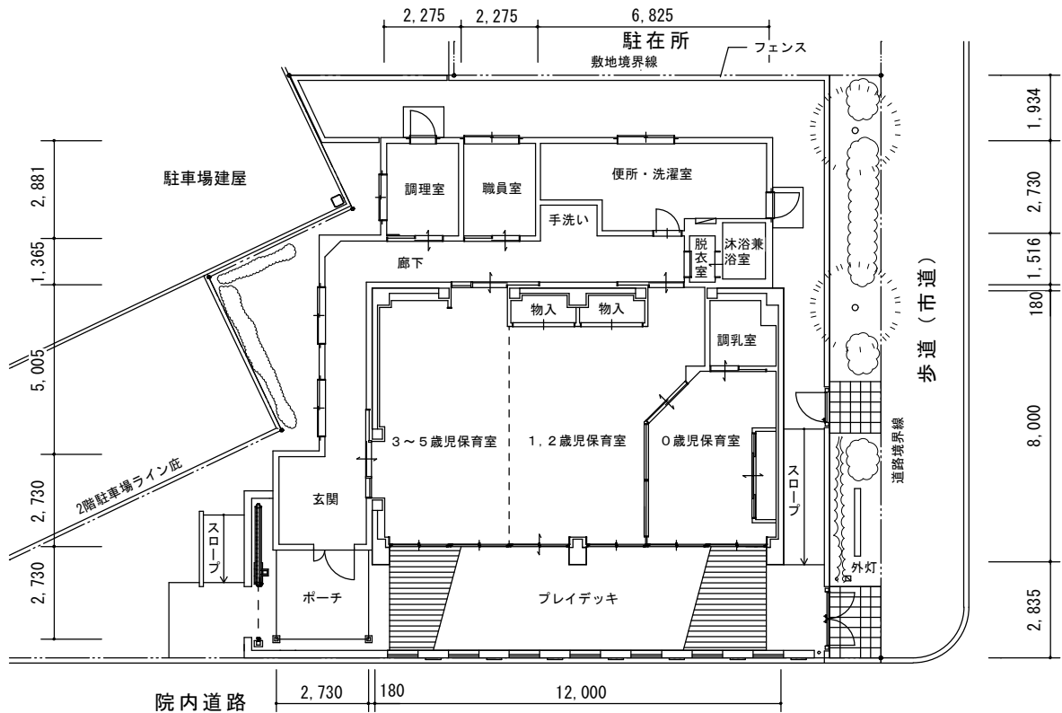
平面図 S=1/200
